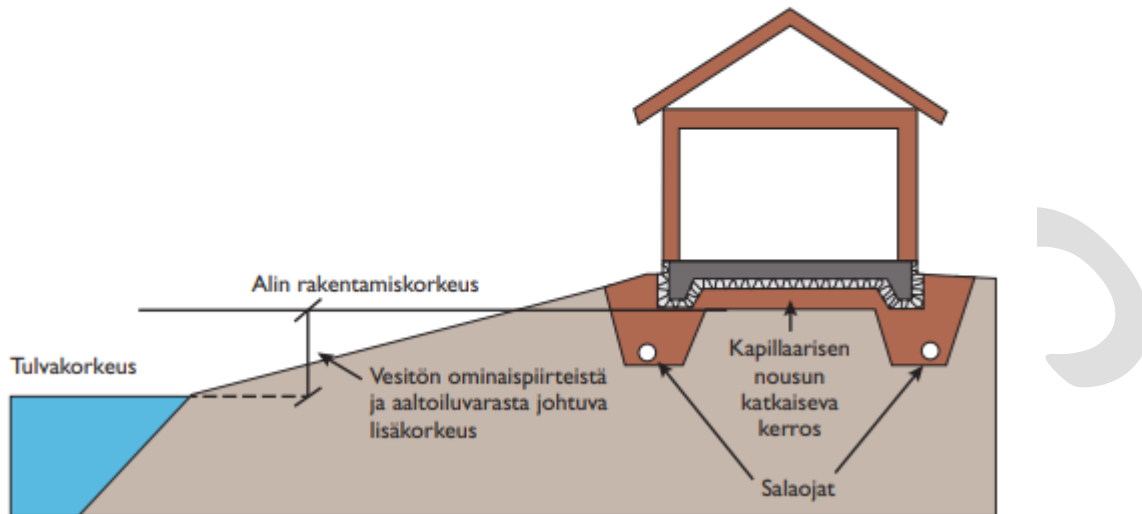
Kuva 2. Alin suositeltava rakentamiskorkeus matalaperustuksella. (Ympäristöopas 2014)
