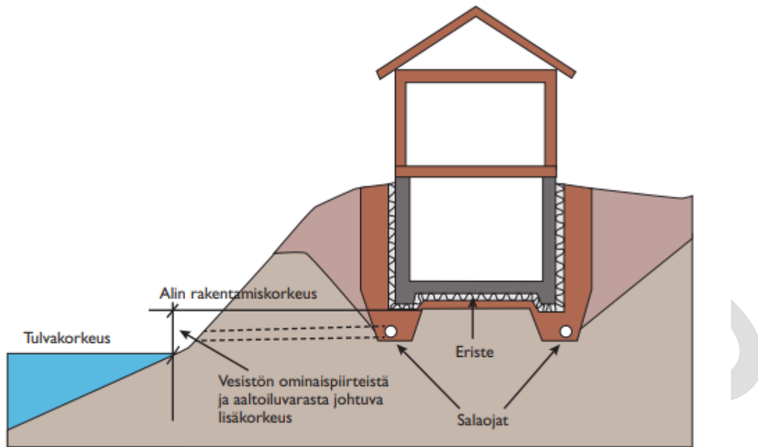
Kuva 4. Alin suositeltava rakentamiskorkeus maanvaraiselle perusmuuriperustukselle kellarilla. (Ympäristöopas 2014)
